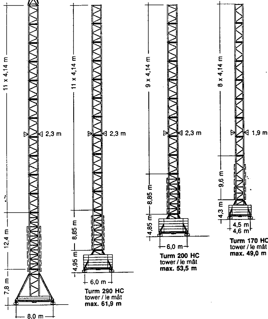
Turm 290 HC tower / le mât max. 68,4 m
